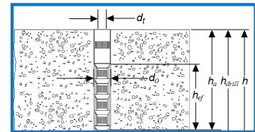
FIGURA 3 - Detalle deinstalacion tipica para insertos internamente roscados
